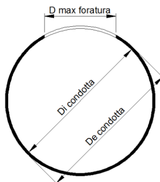
Immagine 2 - Sezione condotta
